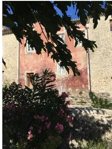
Enduit à pierres vues à gauche et à droite Enduit lisse ou finement taloché au centre
